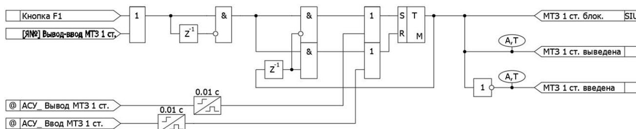
Рисунок К.1 – Функциональная схема алгоритма ввода – вывода функции
