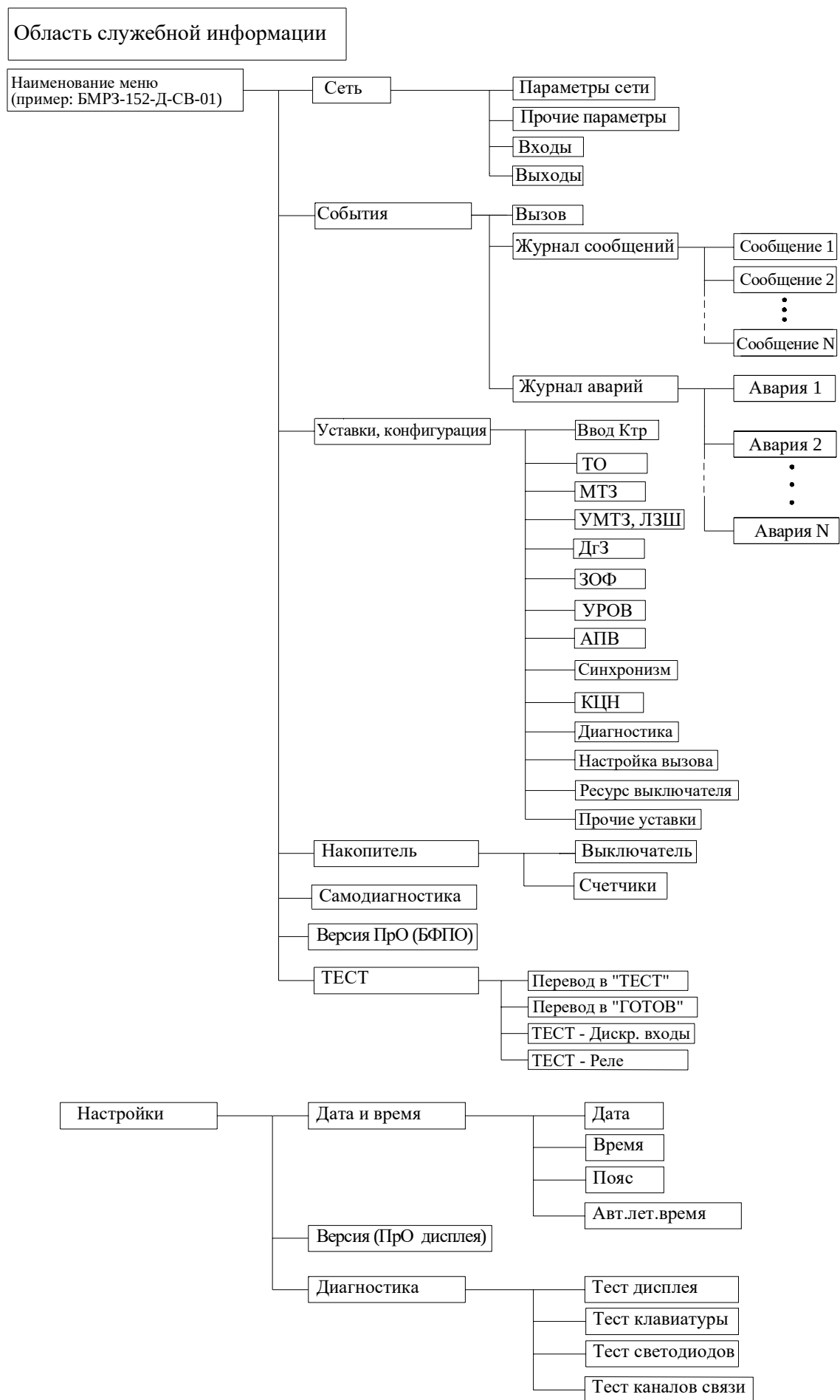
Рисунок А.1 - Пример типовой структуры и содержания пунктов меню монохромного дисплея
