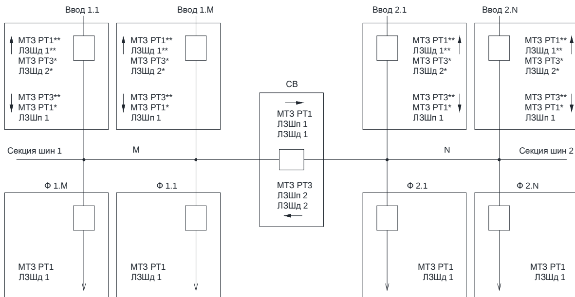
а) структура подстанции и определение направления защит
