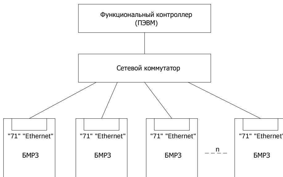
Рисунок В.2 - Организация топологии сети (Ethernet)
