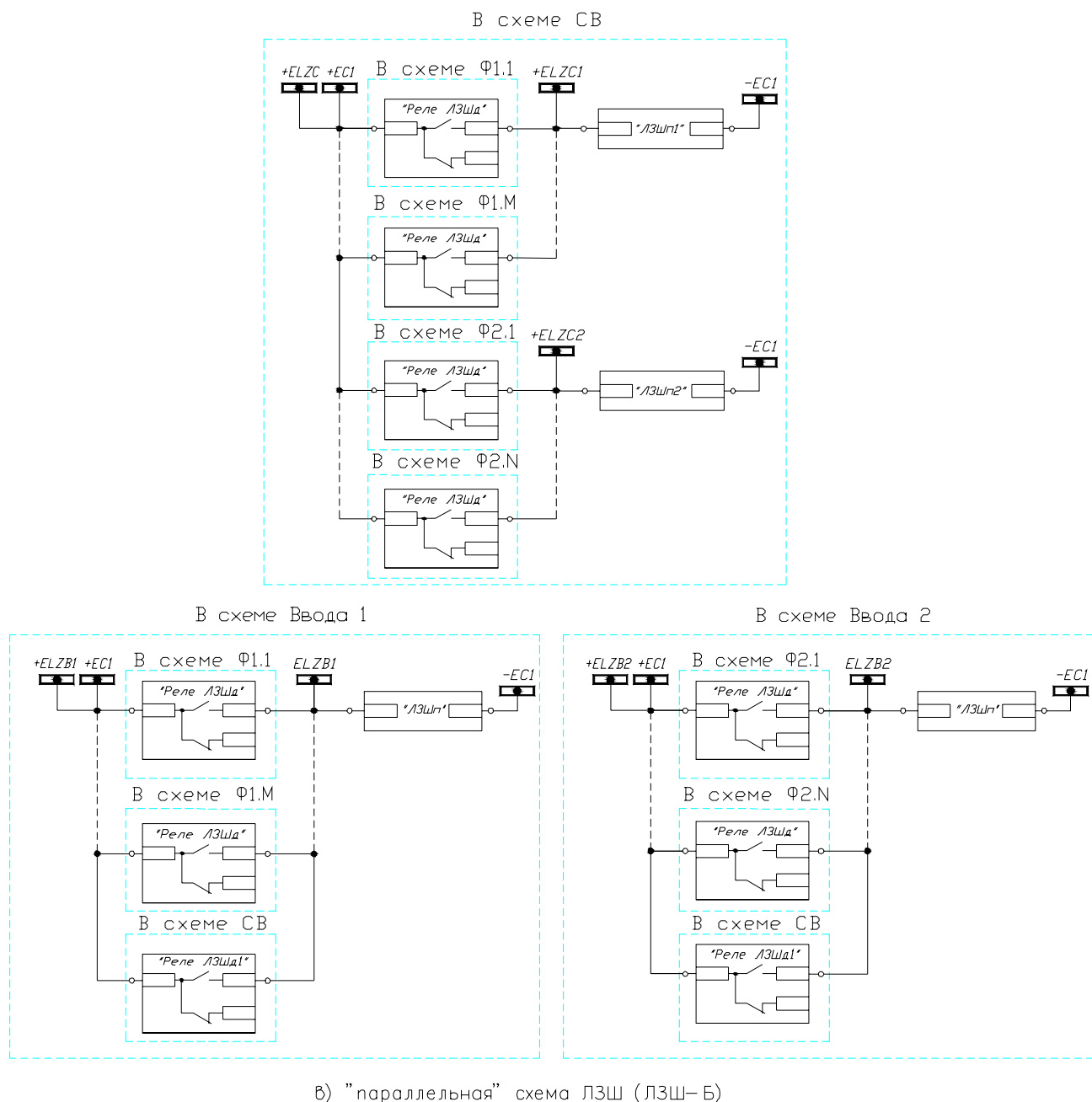
Рисунок И.1 (лист 2 из 2) – Структура ЛЗШ подстанции
