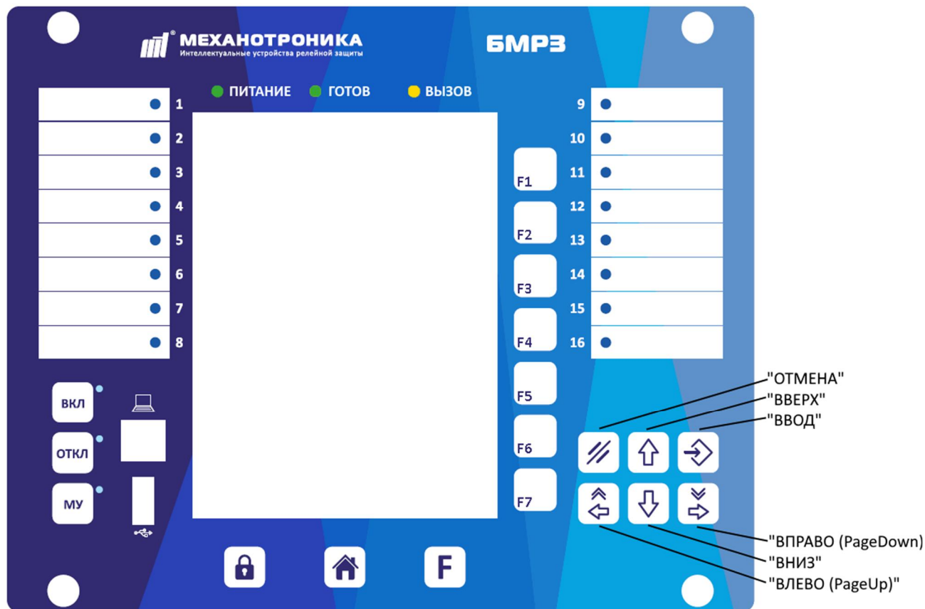
Рисунок 4 – Пример лицевой панели пульта с графическим дисплеем
