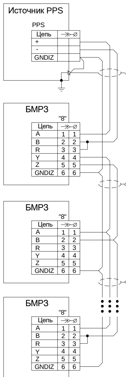
Рисунок В.3 - Схема электрическая подключения цепей PPS (вариант 1)
