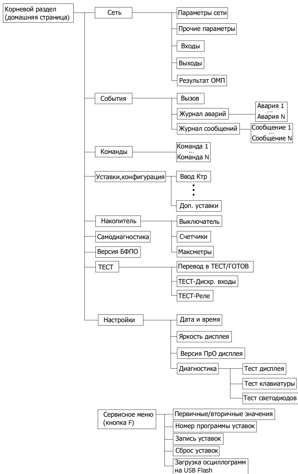
Рисунок А.2 - Пример типовой структуры и содержания пунктов меню графического дисплея
