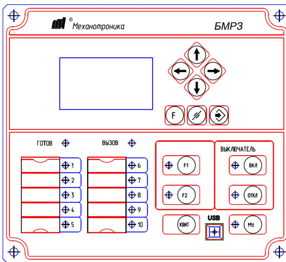
Рисунок 3 – Пример лицевой панели пульта с монохромным дисплеем
