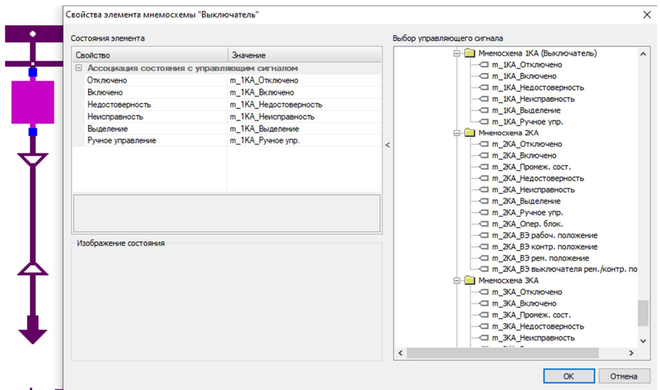
Рисунок Л.1 – Пример ассоциации состояния КА с управляющими сигналами в окне свойств элемента "Выключатель" редактора мнемосхем программного комплекса "Конфигуратор - МТ"
